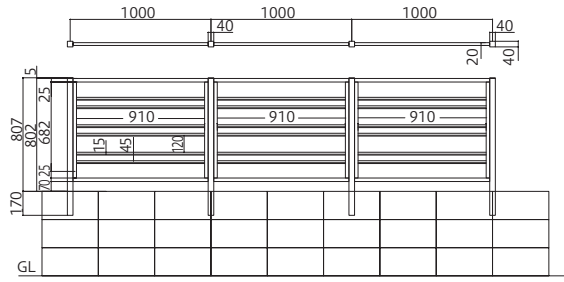
マイティグレインフェンス 2型 (デコII) T-8
