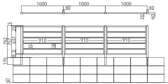
マイティグレインフェンス 1型 (デコII) T-8
