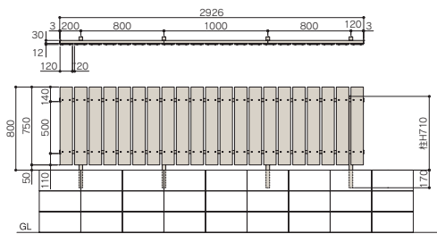
T-8型 (ブロック上に施工した例) タテバリ T-8, H=800 隙間20mm
