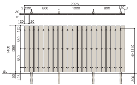
T-14型 ※H1200超はブロック上での施工はできません。 タテバリ T-14, H=1400 隙間20mm
