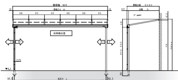
前枠 タイプC ●積雪20cm 間口2.5間×出幅9尺、間口3.0間×出幅6~9尺 ●積雪50cm 間口1.0~2.0間×出幅7~9尺、間口2.5間×出幅3~6尺
