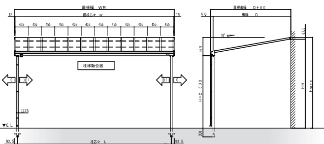
前枠 タイプC
