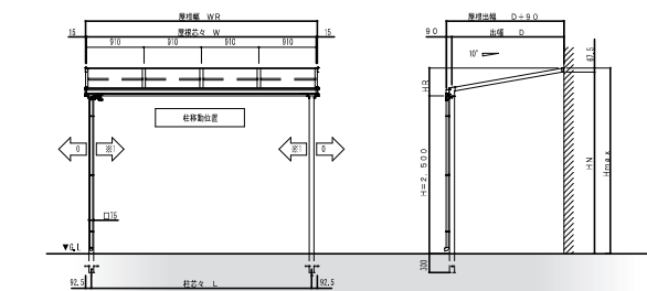
前枠 タイプC
