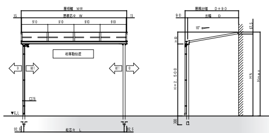
前枠 タイプC ●積雪20cm 間口2.5間×出幅9尺、間口3.0間×出幅6~9尺 ●積雪50cm 間口1.0~2.0間×出幅7~9尺、間口2.5間×出幅3~6尺
